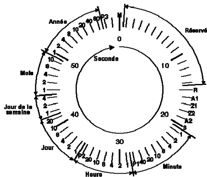
Figure 4 : Trame envoyée par l'émetteur (voir annexe pour détail)
