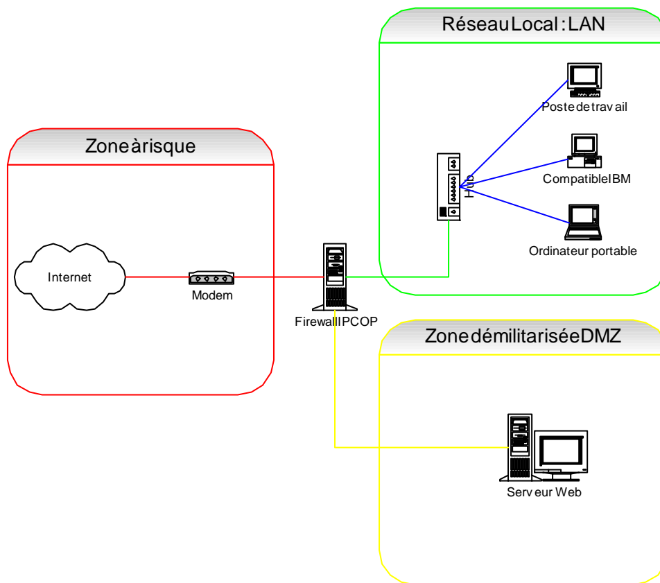
Figure 35 : Modélisation de la DMZ
