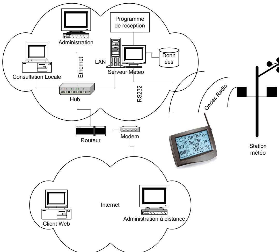
Figure 9 : Schéma implantation
