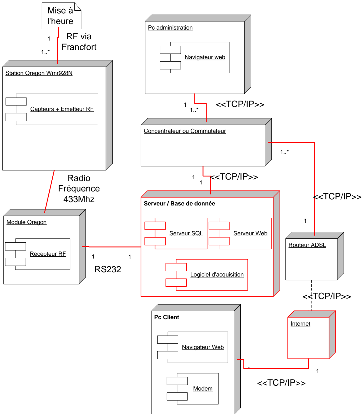
Figure 10 : Diagramme de déploiement
