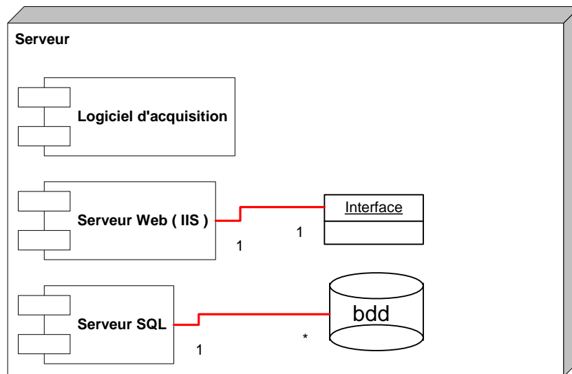
Figure 15: Modélisation
