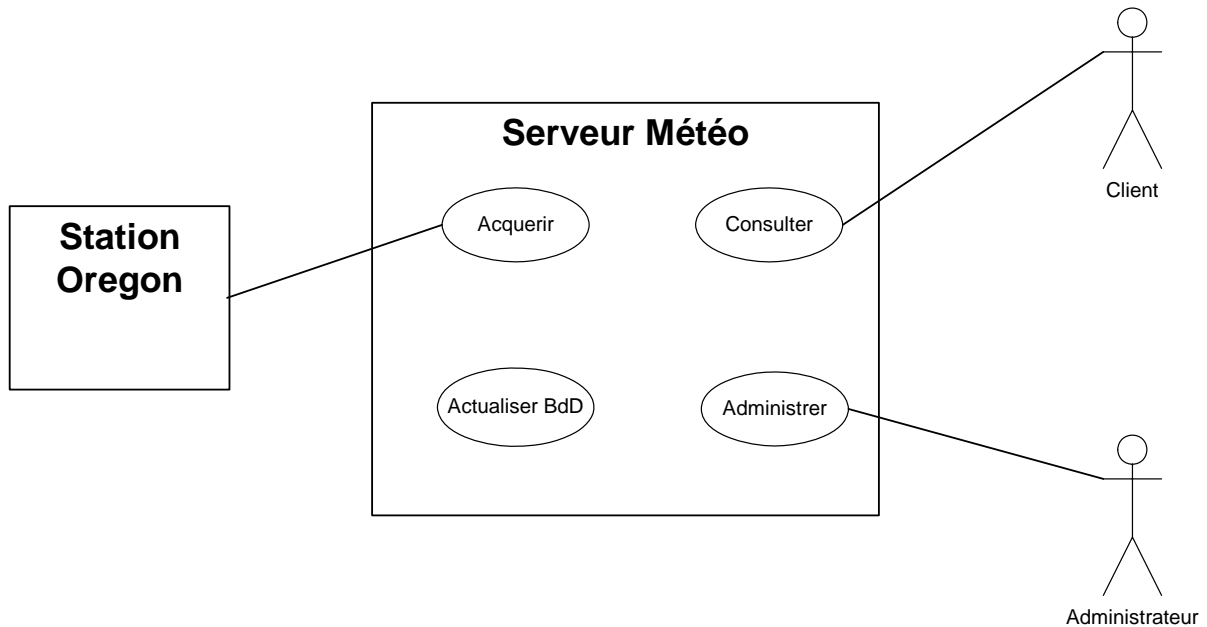
Figure 17 : Cas d'utilisation
