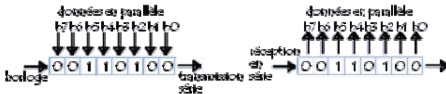
Figure 7 : Sérialisation/Dé sérialisation
